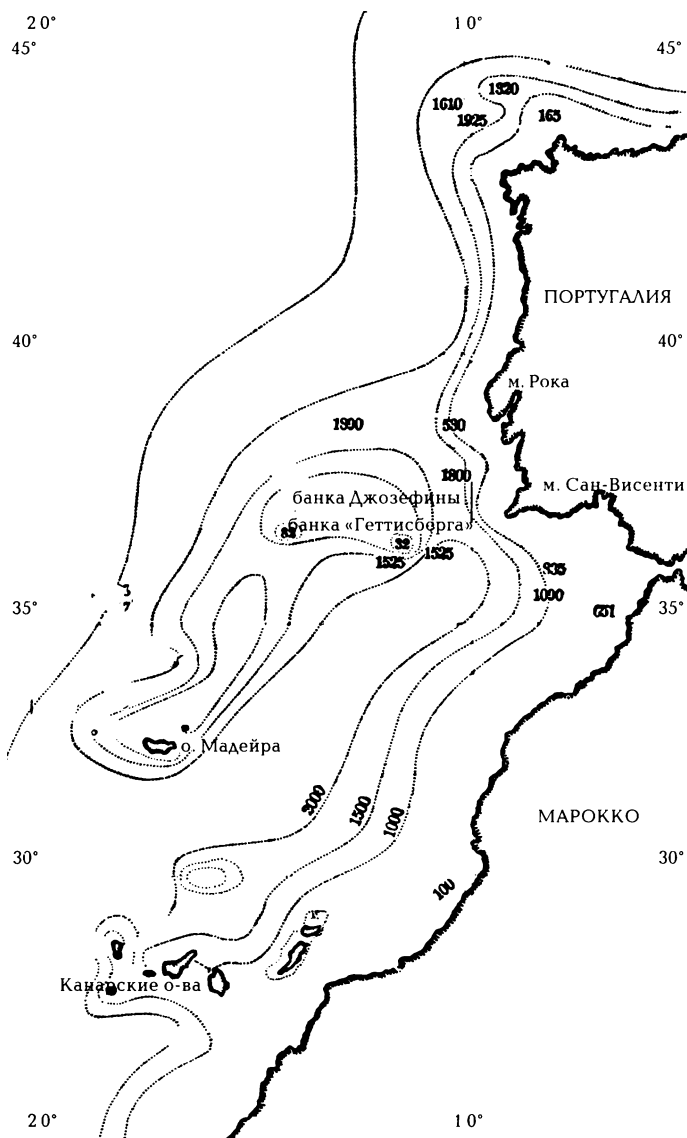
Древние острова между Атлантидой и Средиземным морем по результатам глубоководного зондирования
