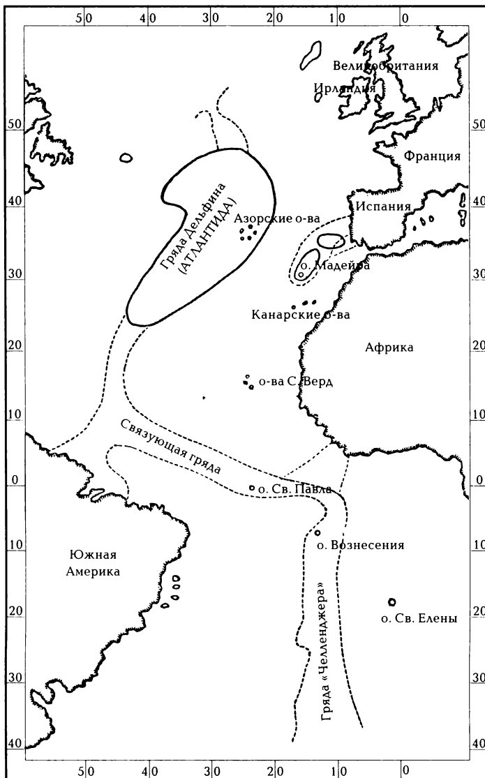
Карта Атлантиды с прилегающими островами и горными хребтами по результатам глубоководного зондирования
