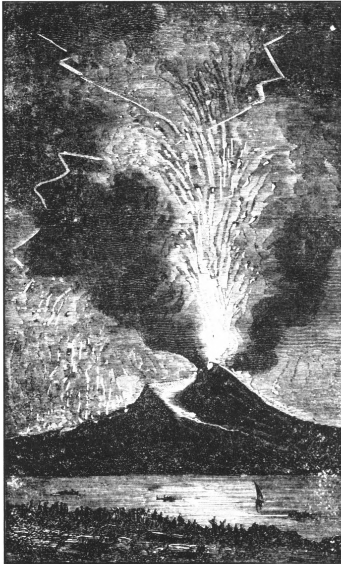
Извержение Везувия в 1737 году
