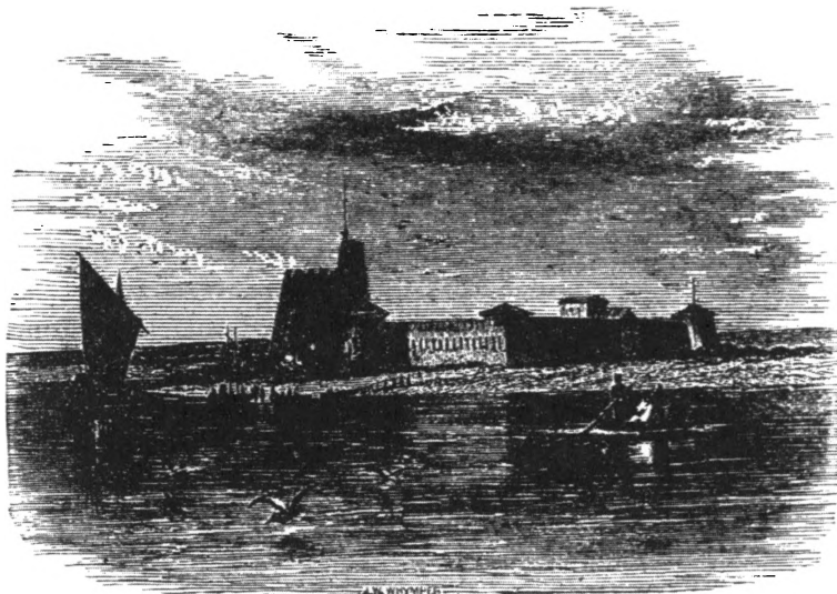
Форт Синдри на восточном рукаве Инда до его затопления во время землетрясения в 1819 году
