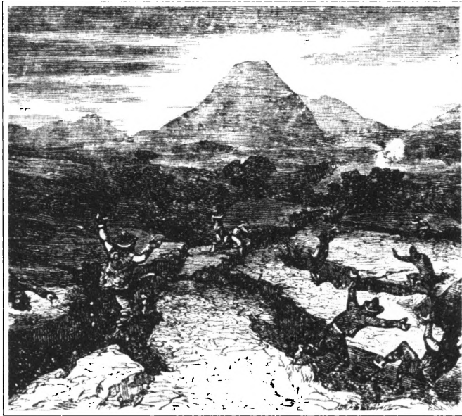
Калабрийские крестьяне, гибнущие в трещинах
