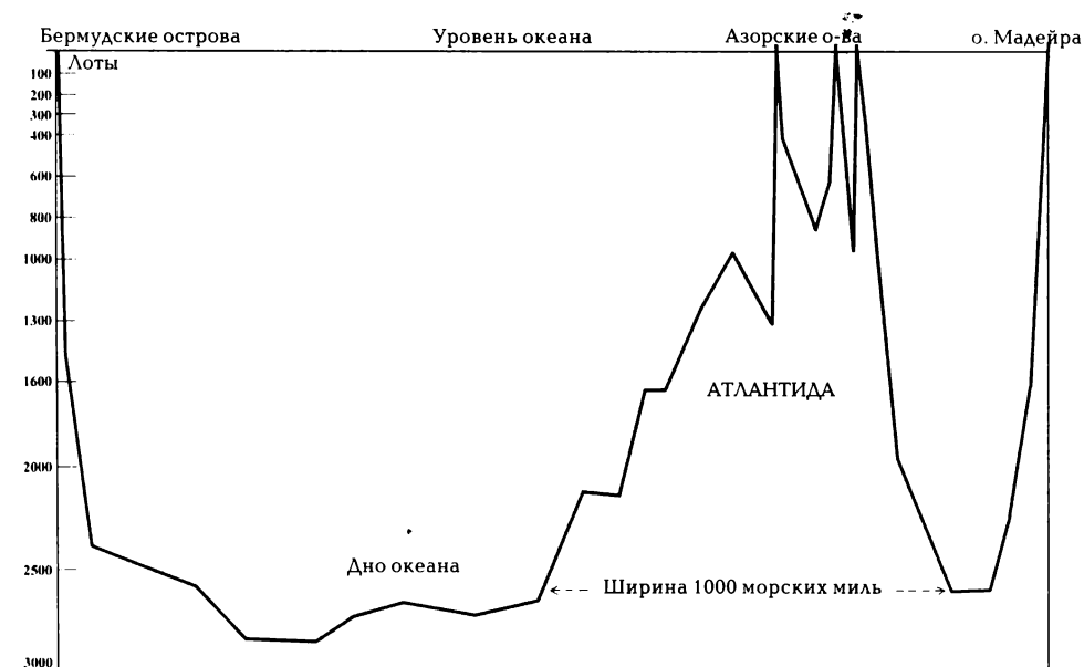
Геологический профиль Атлантиды (получен в ходе глубоководного зондирования с английского корабля «Челленджер» и американского корабля «Дельфин»)
