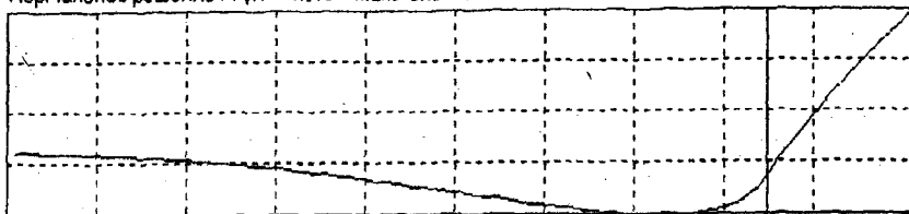
Рис. 2.3. Характер изменения g_{00} для двух близких к пограничному коллапсу случаев - до появления второго внутреннего экстремума ( R/r_1 = 1.1 ) и при наличии такового ( R/r_1 = 1.015 ).
