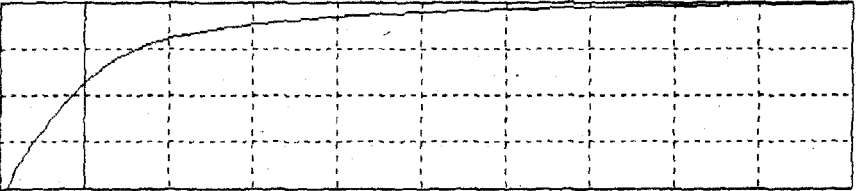
Рис. 2.6. Графики давления и g_{00} при относительно сильном коллапсе ( R/r_1 = 0.1 )
