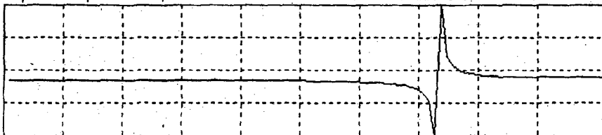
Рис. 2.4. Характер изменения безразмерного давления для двух близких к пограничному коллапсу случаев - до появления второго внутреннего экстремума ( R/r_1 = 1.1 ) и при наличии такового ( R/r_1 = 1.015 ).
