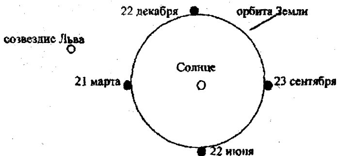
Рис. 4. Расположение Солнца и созвездия Льва относительно Земли
