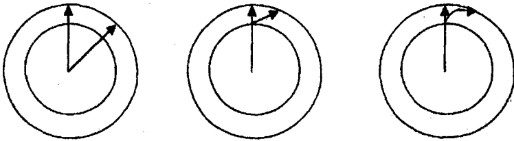
Рис. 1. Эффект “перемещения” точек на поверхности гиперсферы для неподвижных в пространстве объектов (слева), движущихся по инерции (в центре) и ускоренно (справа)
