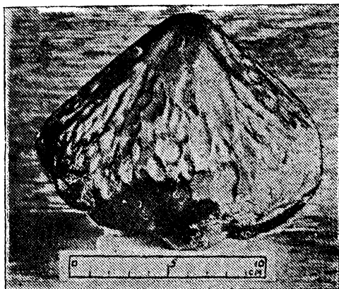
Рис. 13. Метеорит Каракол (хондрит). Упал 9 мая 1840 года в б. Семипалатинской области. Вес 2,79 кг.
