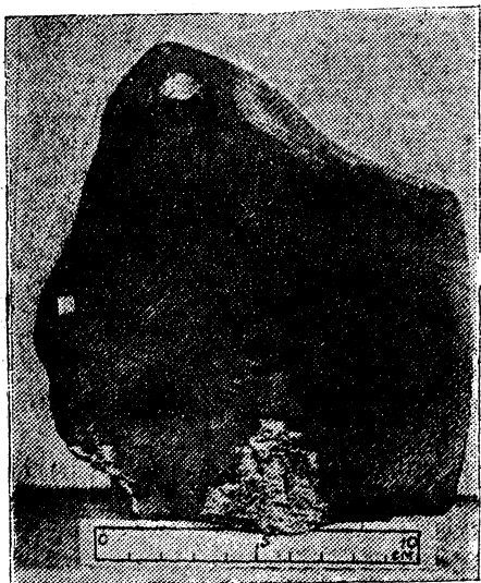
Рис. 12. Метеорит Николаевка (хондрит). Упал 11 июня 1935 года в Павлодарской области. Вес 4,02 кг.
