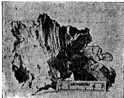
Рис. 4. Осколок Сихотэ Алинского метеорита, извлеченный из кратера.
