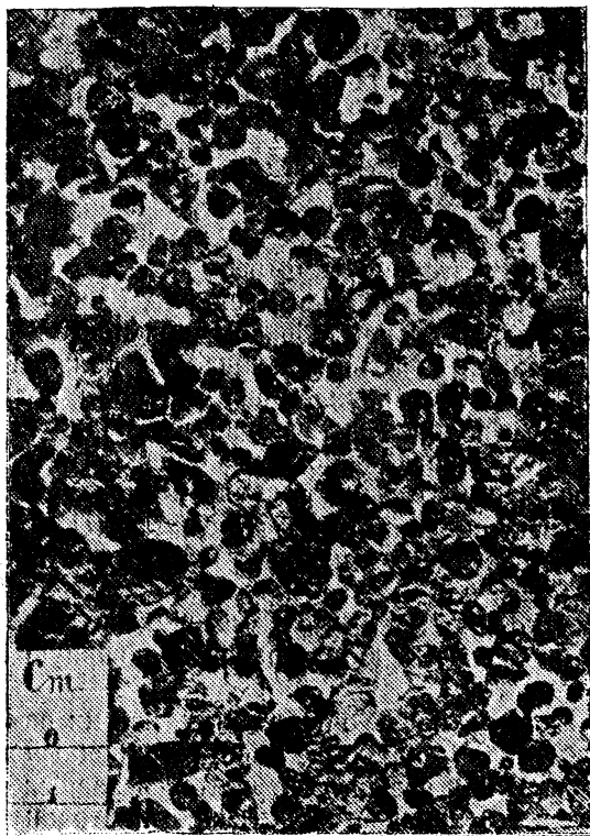
Рис. 11. Палласово железо (внутреннее строение).
