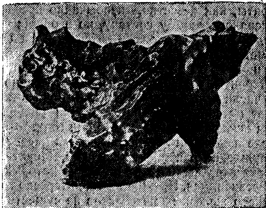
Рис. 9. Балочная структура Сихотэ-Алинского метеорита.
