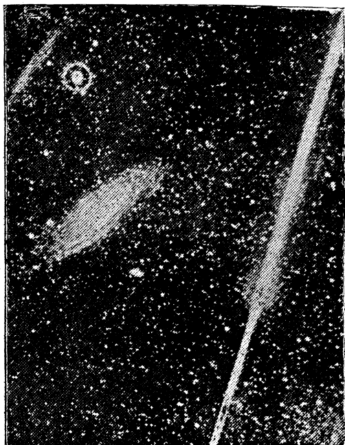
Рис. 6. След метеора в области туманностей Андромеды.
