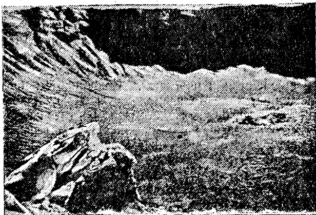
Рис. 5. Аризонский метеоритный кратер (внутренняя часть).
