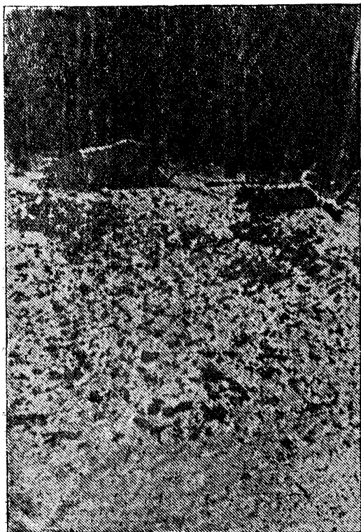
Рис. 3. Внутренний вид кратера, образовавшегося от падения Сихотэ-Алинского метеорита.
