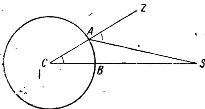
Рис. 16. Измерение Земли.
