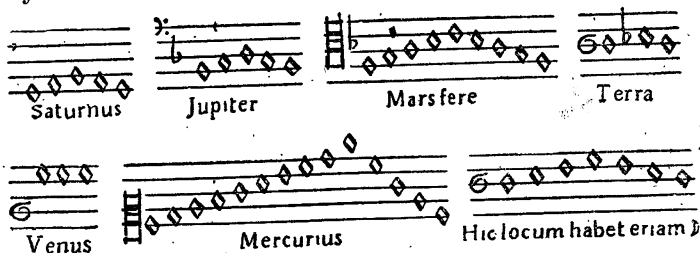
Рис. 60. «Музыка сфер» по Кеплеру. Из Гармонии мира .
