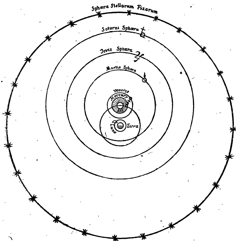
Рис. 50. Система мира Тихо.
