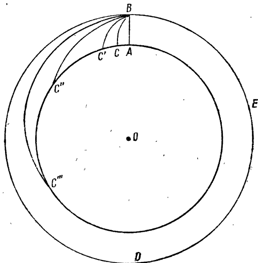
Рис. 69. Луна, рассматриваемая как ядро.
