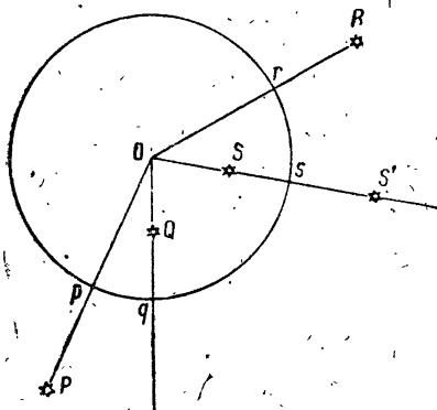
Рис. 1. Небесная сфера.
