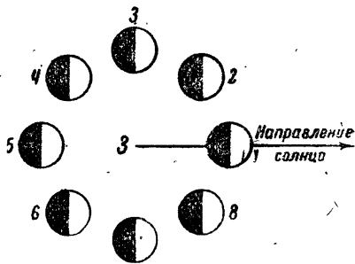
Рис. 10. Фазы Луны.
