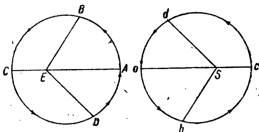
Рис. 37. Относительные движения Солнца и Земли.
