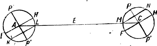
Рис. 40. Коперниково объяснение времён года. Из De Revolutionibus .
