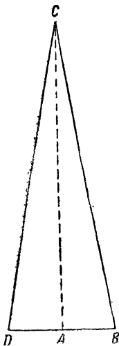
Рис. 72. Абберация света. Из статьи Брайлея.
