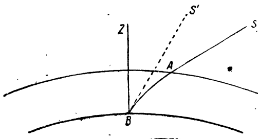
Рис. 32. Атмосферное преломление.
