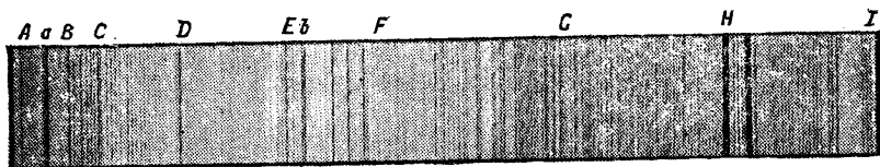
Рис. 94. Фраунгоферова карта солнечного спектра (красный конец спектра слева, фиолетовый справа).
