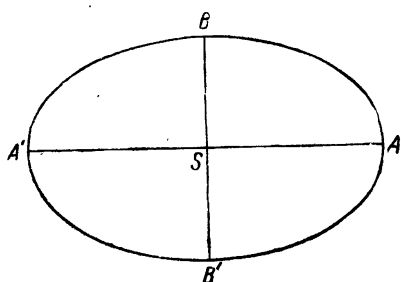
Рис. 74. Аберрационный эллипс.
