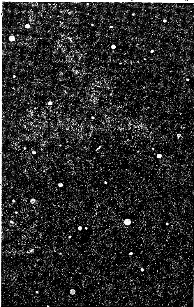
Рис. 85. Фотографический след малой планеты.
