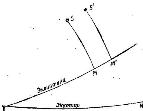
Рис. 21. Возрастание долготы звезды.
