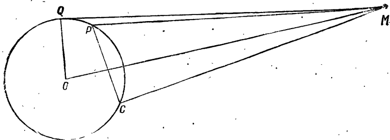
Рис. 67. Параллакс планеты.
