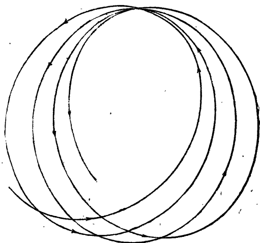
Рис: 79. Варьирующий эллипс.
