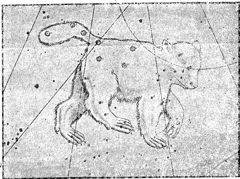
Рис. 5. Большая Медведица. Из Уранометрии Байера (1603).
