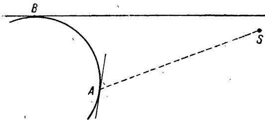
Рис. 12. Кривизна Земли.
