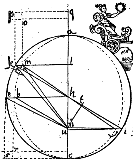
Рис. 59. Диаграмма Кеплера, иллюстрирующая законы планетных движений. Из Комментарий о движениях Марса .
