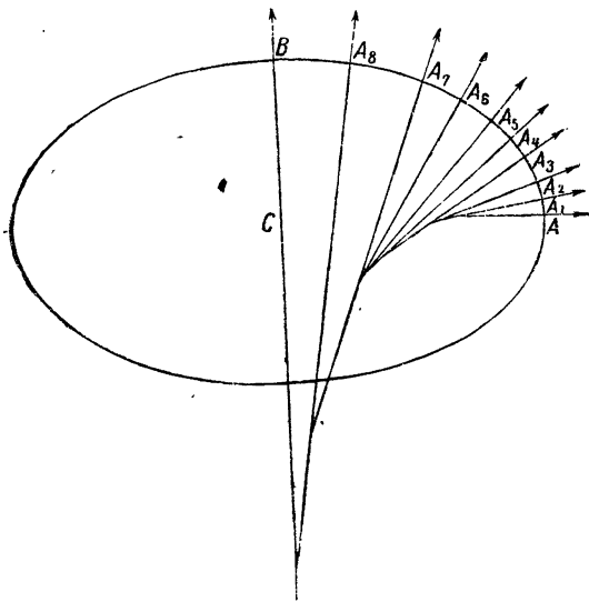
Рис. 76. Изменение кривизны Земли.
