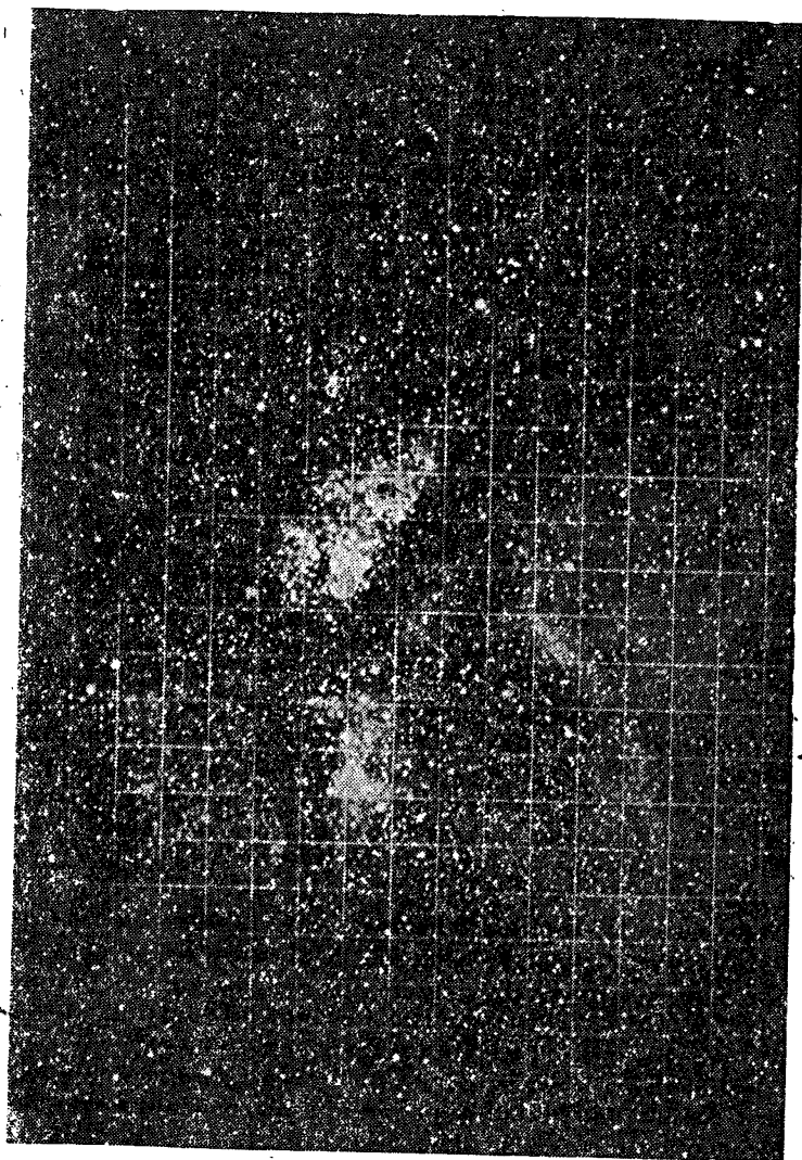
Рис. 97. Туманность около \eta Аргуса. С фотографии Гилла.
