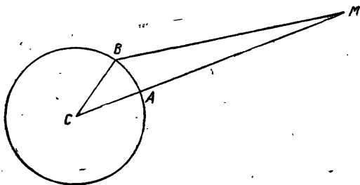
Рис. 31. Параллакс.
