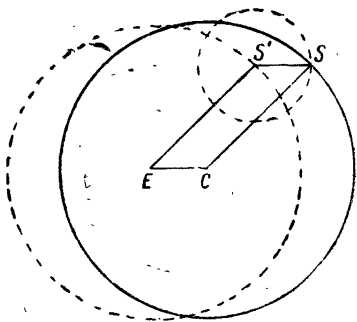
Рис. 19. Эпицикл и деферент.
