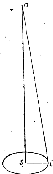
Рис. 84. Параллакс 61 Лебеда.
