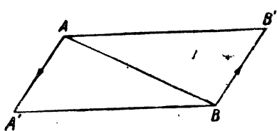
Рис. 36. Относительное движение.
