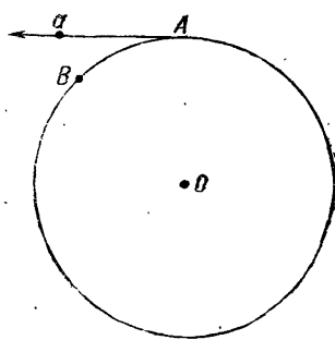
Рис. 68. Круговое движение.
