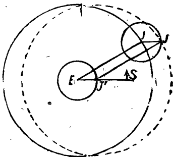
Рис. 43. Эпицикл Юпитера.
