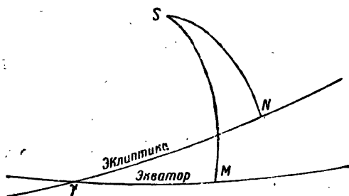
Рис. 14. Экватор и эклиптика.
