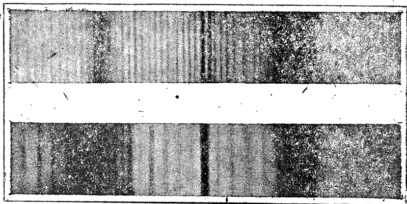
Рис. 100. Спектр \beta Возничего, показывающий линию K в простом и удвоенном виде. С фотографии, снятой в Гарварде.
