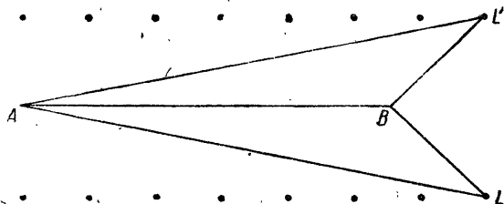
Рис. 82. Иллюстрации к движению Солнца в пространстве.
