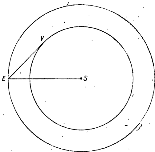
Рис. 41. Орбиты Венеры и Земли.
