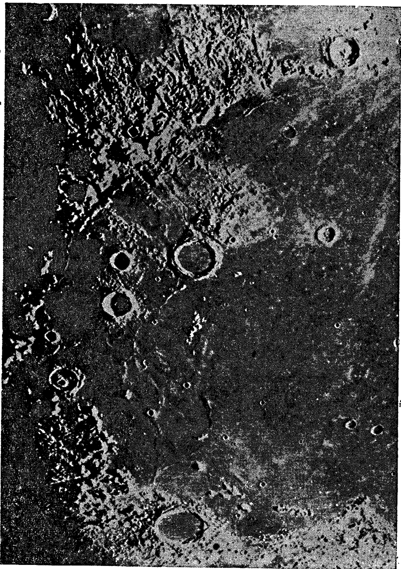
Рис. 91. Апеннины и смежные области Луны; с фотографии Парижской обсерватории.
