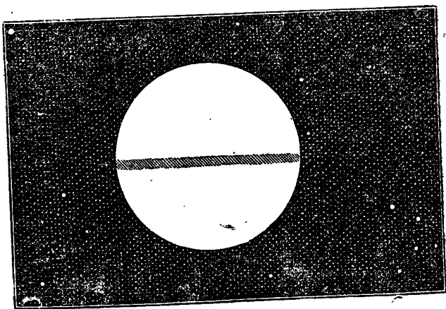
Рис. 63. Сатурн и кольцо, видимое с края. Из Системы Сатурна .
