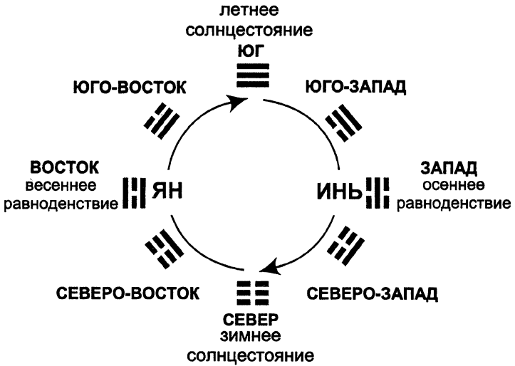
Рис. 7. Стороны света в графическом выражении “Книги Перемен”
