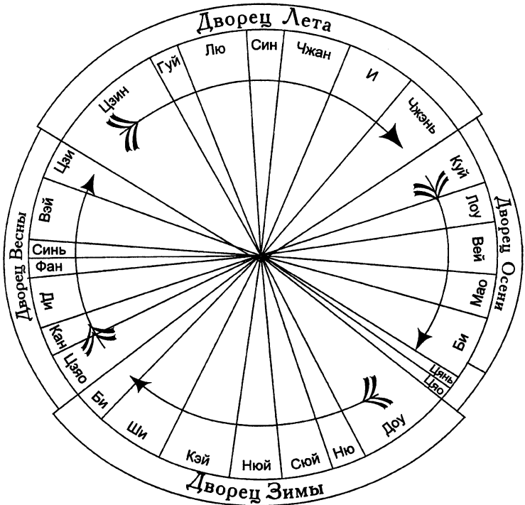
Рис. 4. Полный оборот Солнца в поступательном направлении
