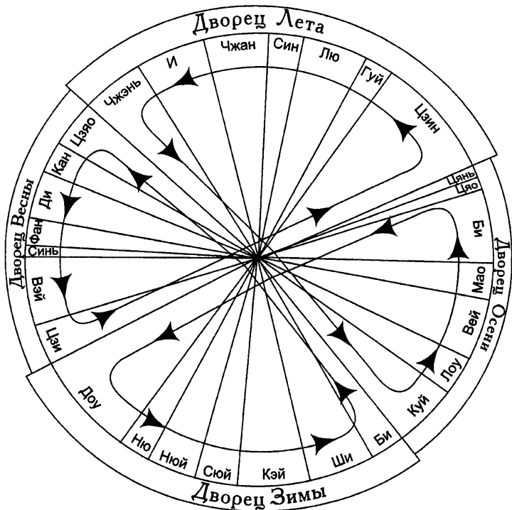
Рис.5. Полный (циклический) оборот Луны и Солнца
