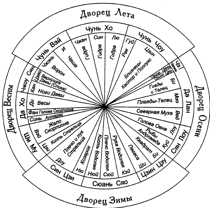
Рис.9. 12-теричные циклы Дворцов времен года
