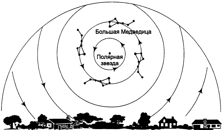
Рис. 6. Вращение Большой Медведицы и звезд вокруг Полярной звезды
