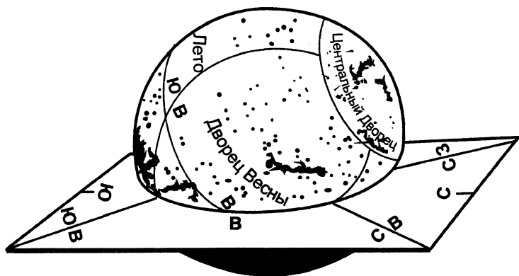
Рис.2. Дворцы времен года
