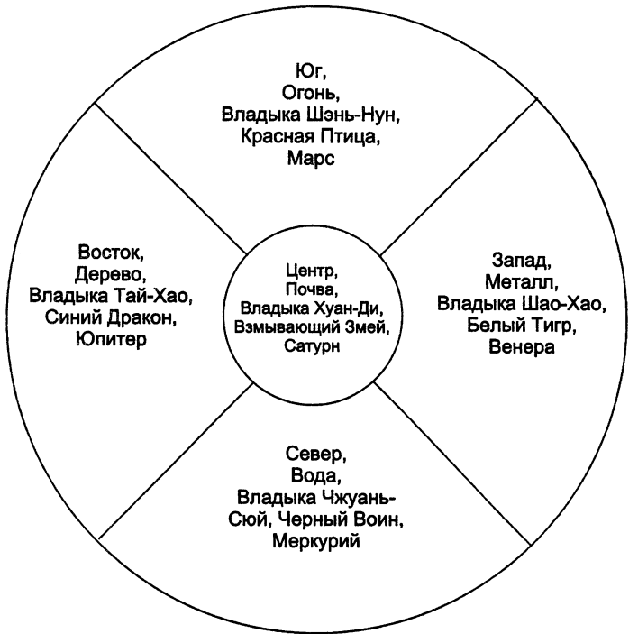
Рис. 8. Аспекты закона Подобия
