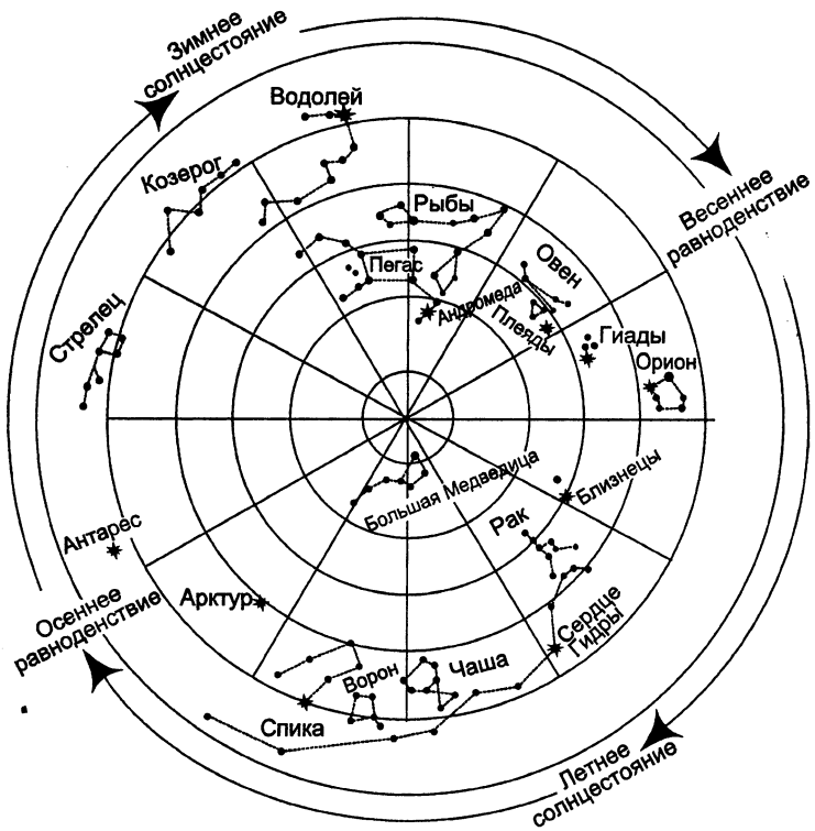
Рис.1. Четыре части света, соответствующие равноденствиям и солнцестояниям
