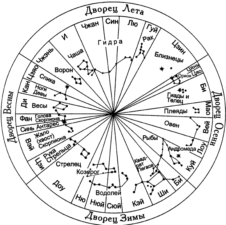
Рис.3. Дворцы времени года и 28 китайских зодиакальных созвездий
