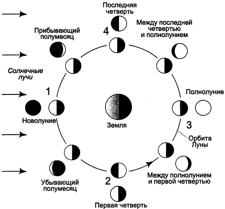
Рис.10. Динамика фаз Луны
