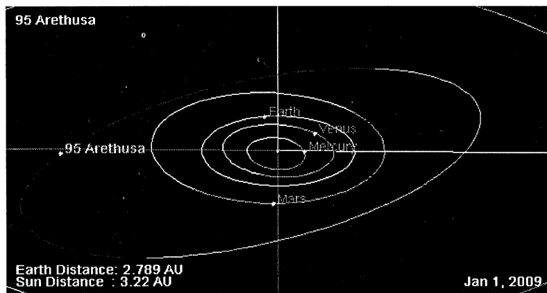
Орбита астероида Аретуза, и его положение в Солнечной системе на 01.01.2009 г. (Рисунок NASA JPL Small Body Orbit)
