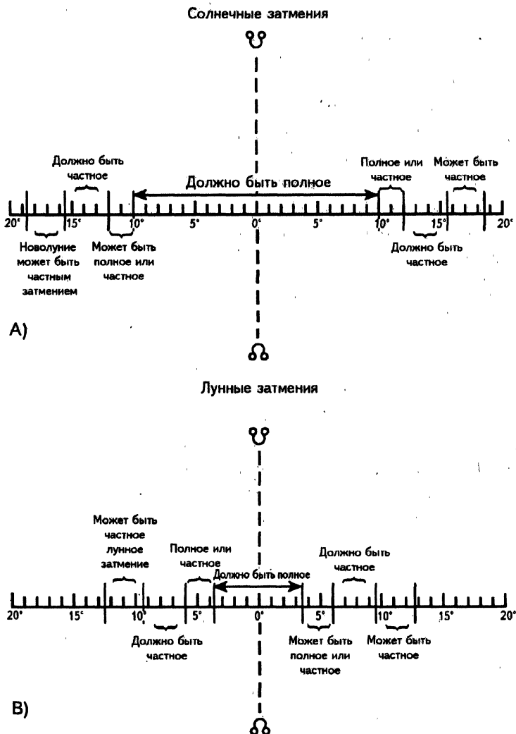
Рис. 40. Данные графики показывают орб Лунного узла, в пределах которого могут происходить солнечные (A) и лунные (B) затмения.
