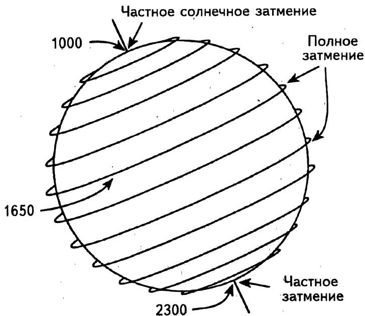
Рис. 45. Цикл сароса,двигающийся с Северного полюса к Южному.
