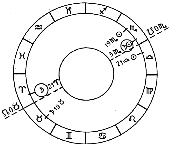
Рис. 42. Полнолуние, дающее лунное затмение, за которым через 14 дней в новолуние будет солнечное затмение.
