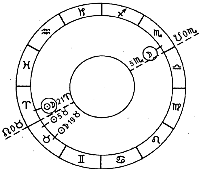
Рис. 41. Новолуние, дающее солнечное затмение, за которым через 14 дней в полнолуние следует лунное затмение.
