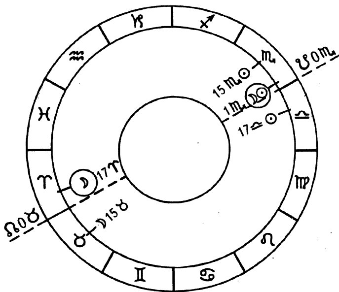
Рис. 43. Полнолуние, не дающее лунного затмения, за которым через 14 дней в новолунии следует солнечное затмение.
