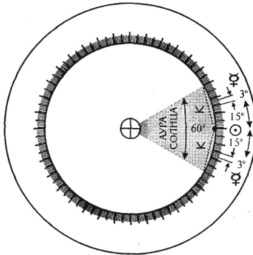
Рис. 9.3. Нейтралы в ауре Солнца
