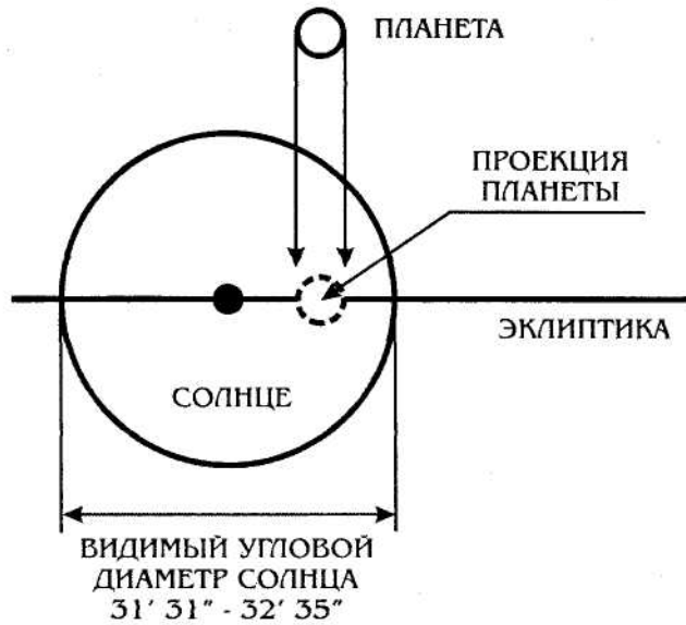
Рис. 9.1. Планета в сердце Солнца
