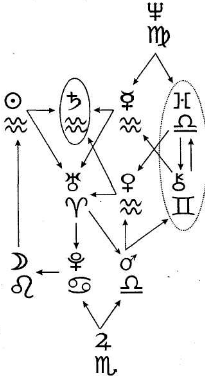
Рис. 4.2. Схема диспозиций
