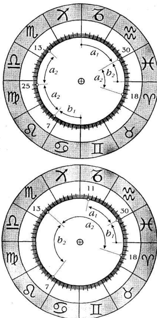
Рис. 12.14. Некоторые Золотые соотношения
