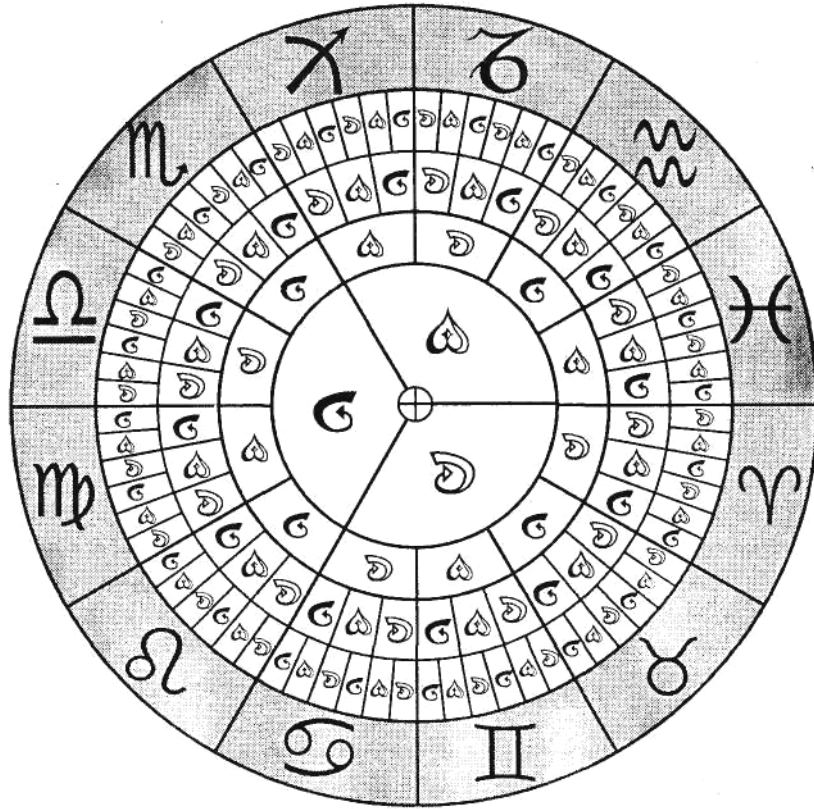
Рис. 12.17. Звезда терм и декада с началами
