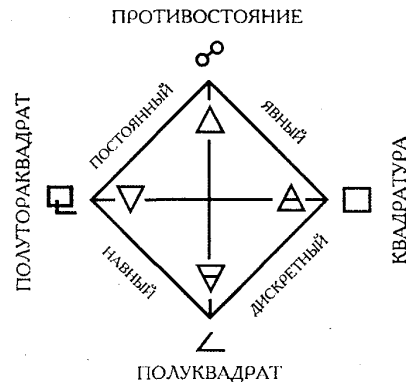
Рис. 3.5. Кватернер аспектов действия
