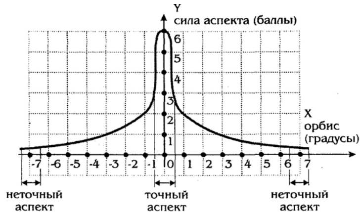
Рис. 2.2. Зависимость силы аспекта от величины орбиса
