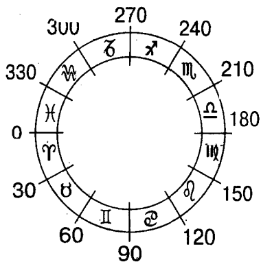
Рис. 4 Градусный круг Зодиака.
