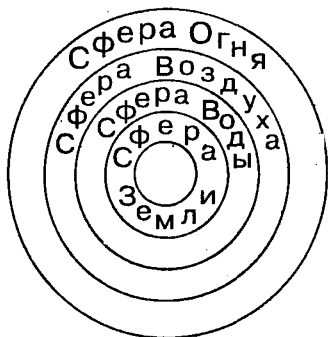
Рис. 7. Сферы четырёх стихий в системе мира Птолемея.
