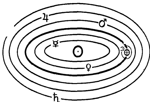
Рис. 24. Схема солнечной системы (планеты септенера).
