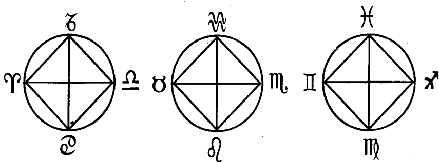
Рис. 8. Кресты: а - кардинальный; б - фиксированный; в - мутабельный.
