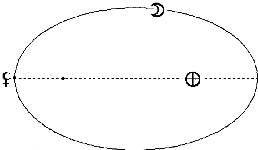
Рис. 3.1. Орбита Луны.
