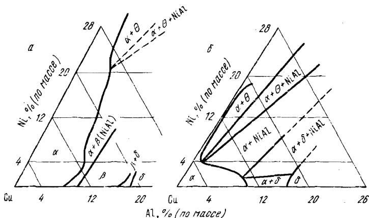
Рис. 16. Изотермическое сечение диаграммы состояния системы медь — алюминий — никель при 1000 (а) и 400 °C (б)
