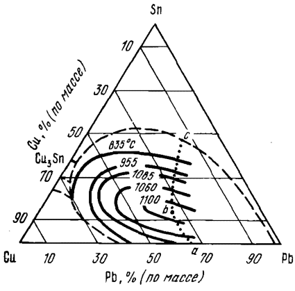
Рис. 27. Диаграмма состояния сплавов системы медь — олово — свинец
