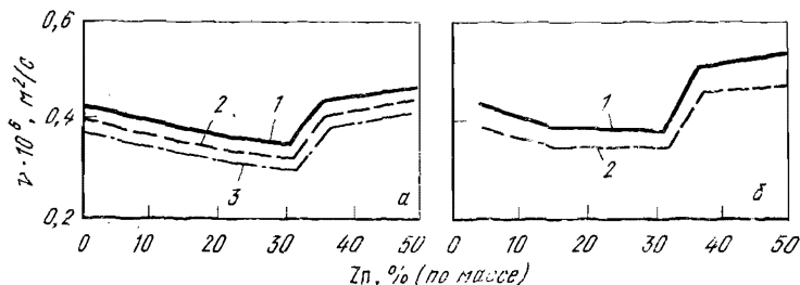
Рис. 54. Кинетическая вязкость расплавов медь — цинк [39]: а — η при температуре 1373 (1), 1423 (2), 1473 К (3); б — η при равных перегревах над T_{лик} , составляющих 323 (1) и 373 К (2)
