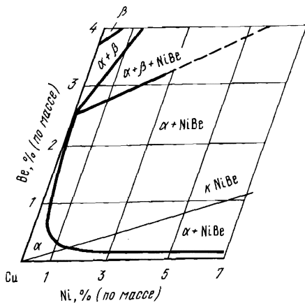
Рис. 19. Изотермическое сечение диаграммы состояния системы медь — бериллий — никель при 820 °С
