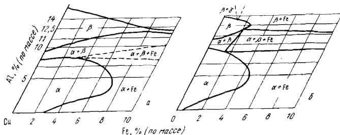
Рис. 14. Изотермическое сечение диаграммы состояния системы медь — алюминий — железо при 1000 (а) и 700 °С (б)
