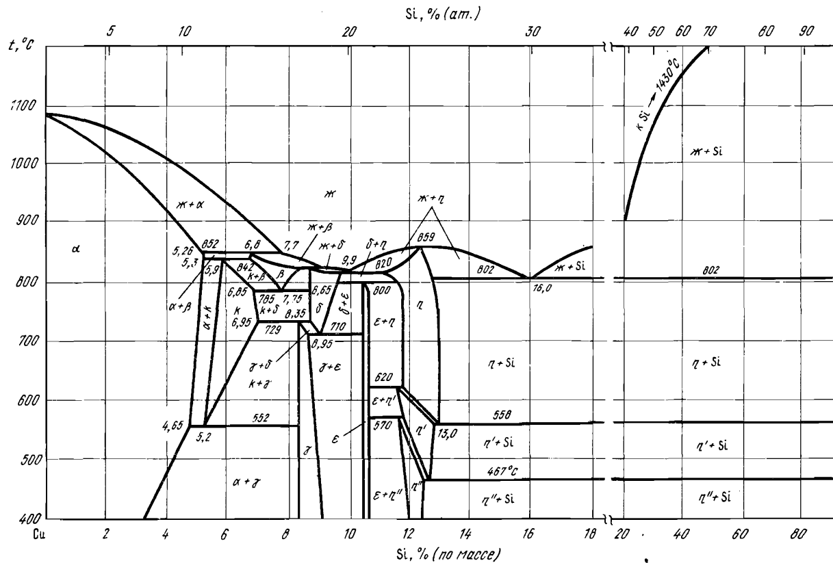
Рис. 5. Диаграмма состояния сплавов системы медь — кремний
