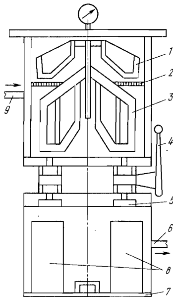
Рис. 85. Установка для вибровакуумирования литейных форм:
