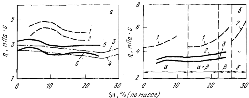
Рис. 53. Динамическая вязкость расплавов медь — олово: а — η при температуре 1273 (1, 3, 5) и 1473 К (2, 4, 6) по данным [37] (1, 2), [38] (3, 4), [39] (5, 6); б — η при равных перегревах над T_{лик} , составляющих 323 (1, 2) и 373 К (3) по данным [37] (1) и [39] (2, 3)
