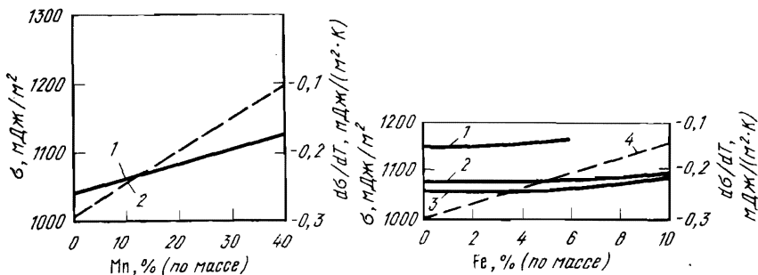
Рис. 48. Поверхностное натяжение (1) и его температурный коэффициент (2) сплавов системы медь — марганец
