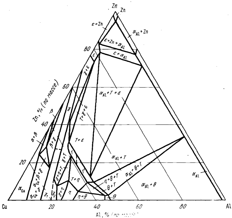
Рис. 18. Изотермическое сечение диаграммы состояния системы медь — алюминий — цинк при 350 °С
