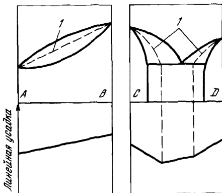
Рис. 67. Кривые линейной усадки сплавов систем A–B и C–D в зависимости от типа диаграммы состояния ( l — линия начала линейной усадки)
