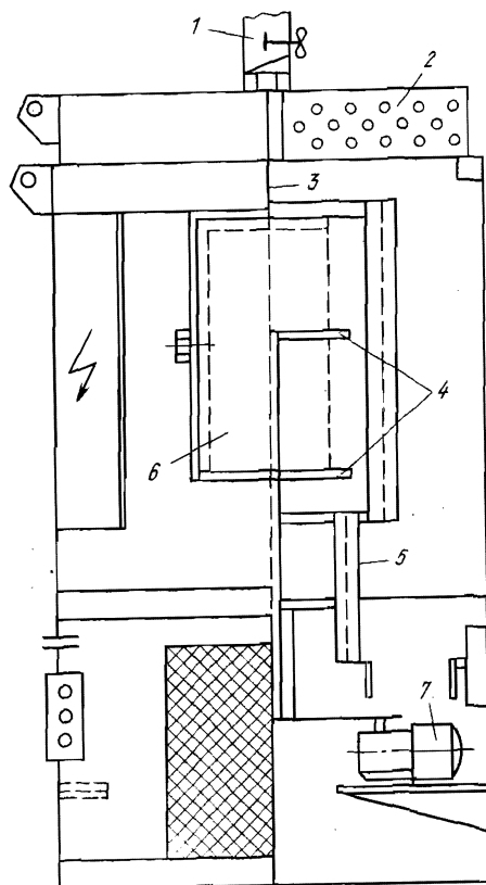
Рис. 88. Схема карусельной печи для прокаливания опок: 1— труба для отвода газов; 2— свод печи с теплоизоляцией; 3— термопара; 4— вращающийся металлический поддон; 5— труба для вытекания расплавленного воска; 6— загрузочное окно; 7— электродвигатель для вращения поддонов
