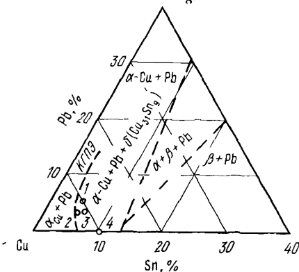
Рис. 71. Медный угол диаграммы состояния сплавов системы \text{Cu} - \text{Sn} - \text{Pb} :
