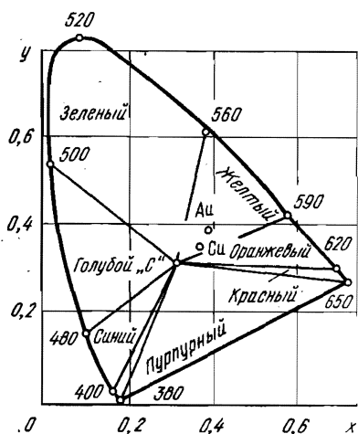
Рис. 79. Цветовой график x, y МКО1931 г. (1 — сплав ZlCrM 583-80 )
