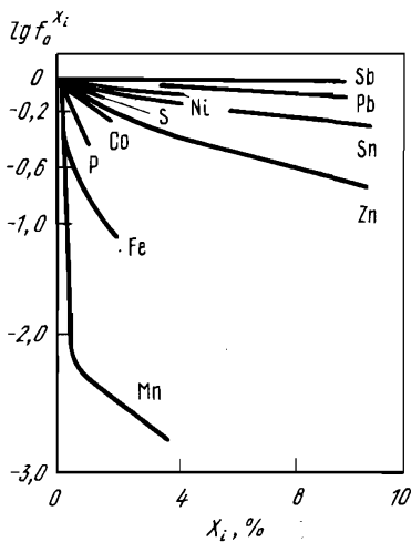
Рис. 37. Влияние элементов X_i на активность кислорода в меди при 1423 К
