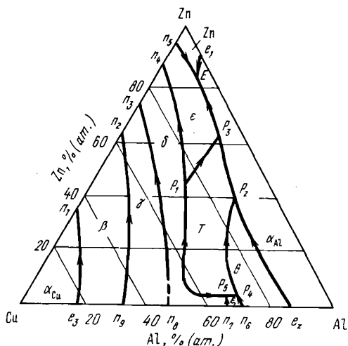
Рис. 17. Проекция поверхности ликвидуса диаграммы состояния систем медь — алюминий — цинк
