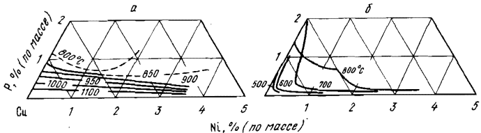
Рис. 26. Изотермы солидуса (а) и растворимости (б) в системе медь — никель — фосфор
