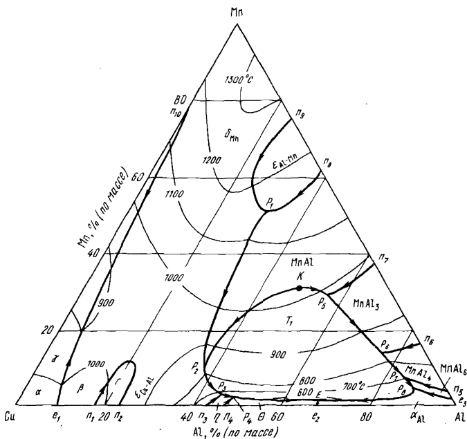
Рис. 15. Проекция поверхностей ликвидуса диаграммы состояния системы медь — алюминий — марганец
