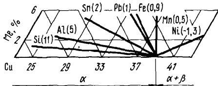
Рис. 72. Влияние легирующих элементов на положение границы между \alpha и \alpha + \beta -областями в системе медь — цинк
