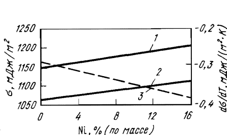
Рис. 47. Поверхностное натяжение при 1473 (1), 1773 К (2) и его температурный коэффициент (3) сплавов системы медь — никель
