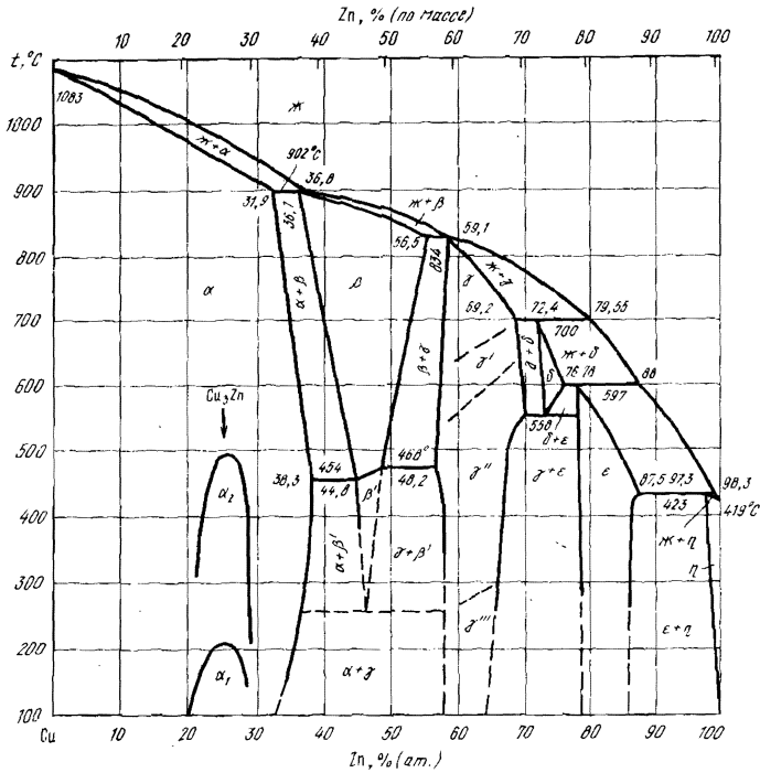
Рис. 13. Диаграмма состояния сплавов системы медь — цинк
