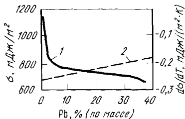
Рис. 44. Поверхностное натяжение при 1473 К (1) и его температурный коэффициент (2) сплавов системы медь — свинец
