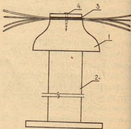
Рис. 54. Шаблон: 1 - шляпа «болванчика», 2 - стойка, 3 - фанерный кружок для прижима сплетенного дна, 4 - шуруп.
