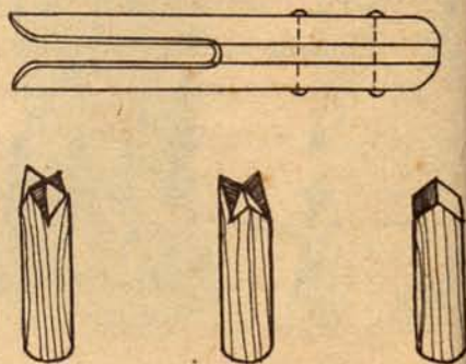
Рис. 2. Инструмент; сверху – зажим (щемила), внизу – щепало для раскалывания прутьев на 2, 3, 4 части.
