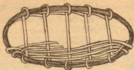
Рис. 46. Отдельно сплетенное дно.
