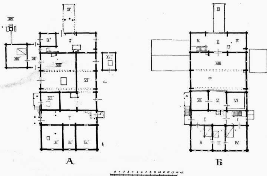
Рис. 5. Схематический план дома б. М. Коровина в Суре.
