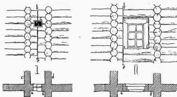
Рис. 6. Типы окон в „заулке“
