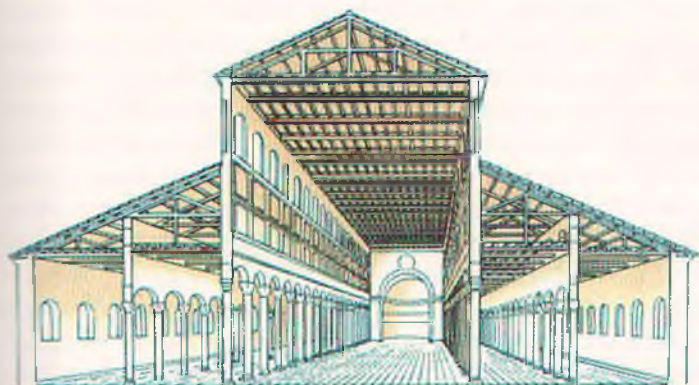
9. Церковь Сан Паоло фуори ле мура в Риме, IV в. Схема поперечного разреза базилики
