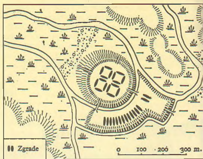
116. Военный лагерь в Треллеборге, Дания, X—XI вв. Реконструкция
