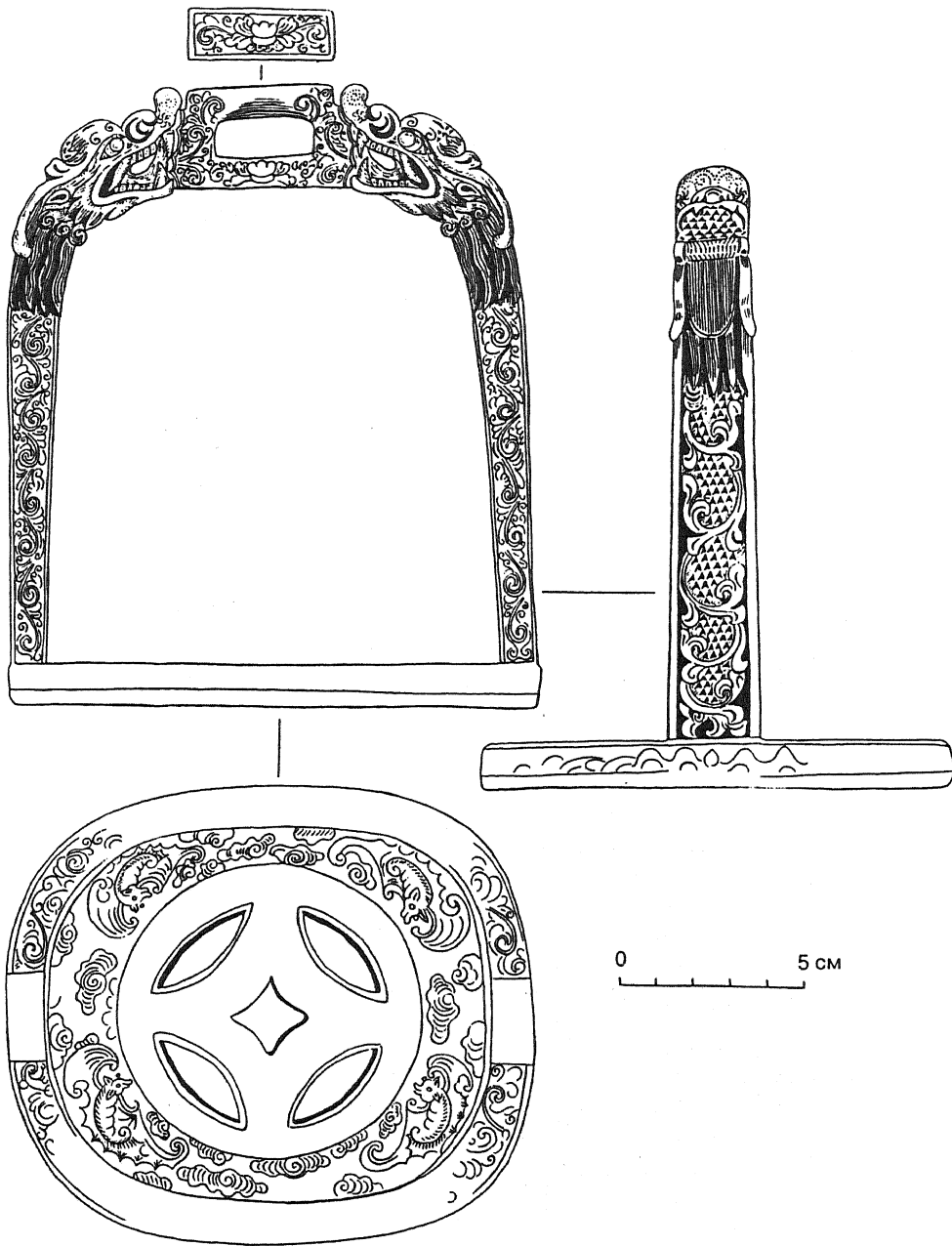
Рис. VI. Стальное стремя
