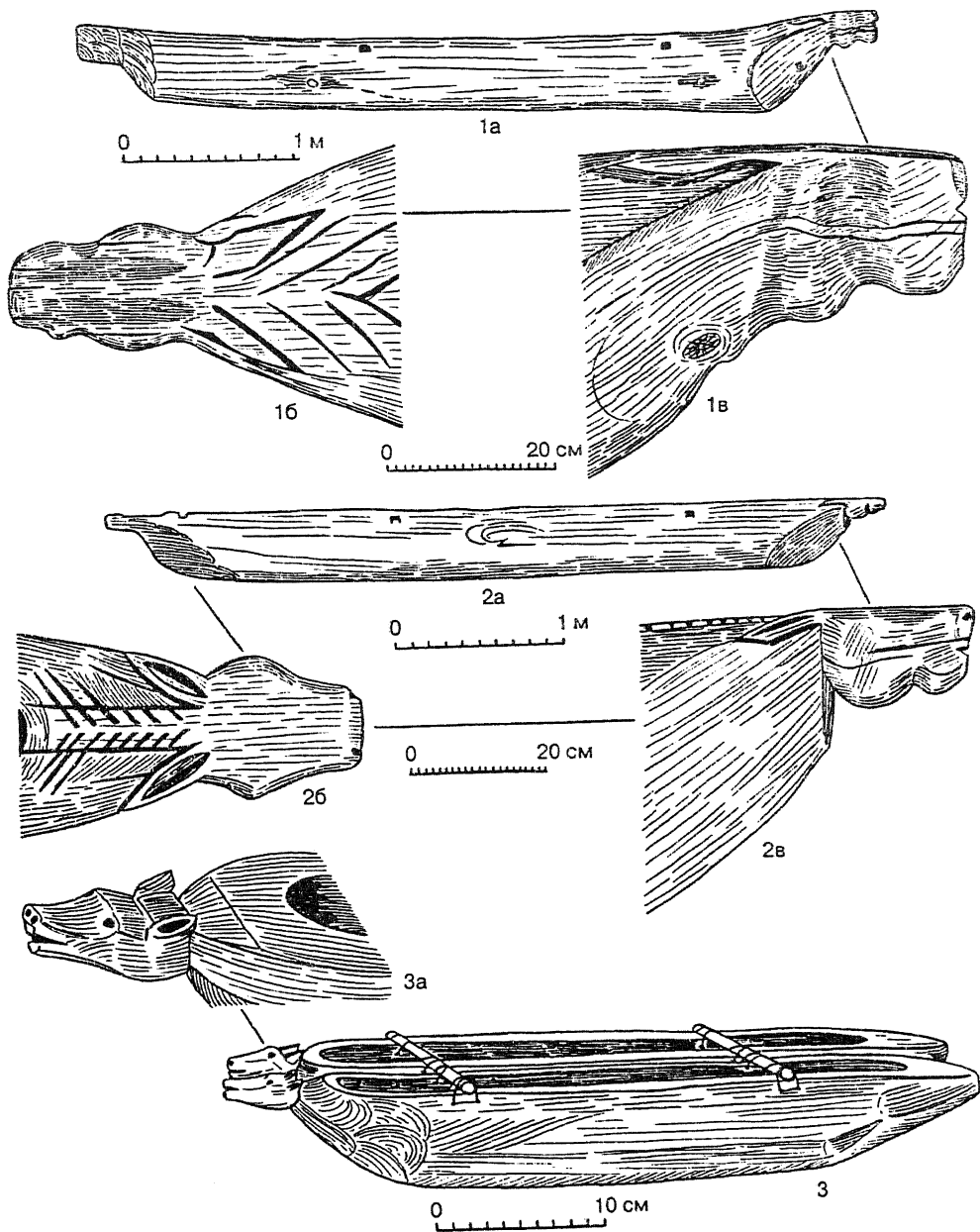
Рис. LVII. Монгольский паром-катамаран гуй онгоц (1, 2) и тувинская модель парома онгоча (3)
