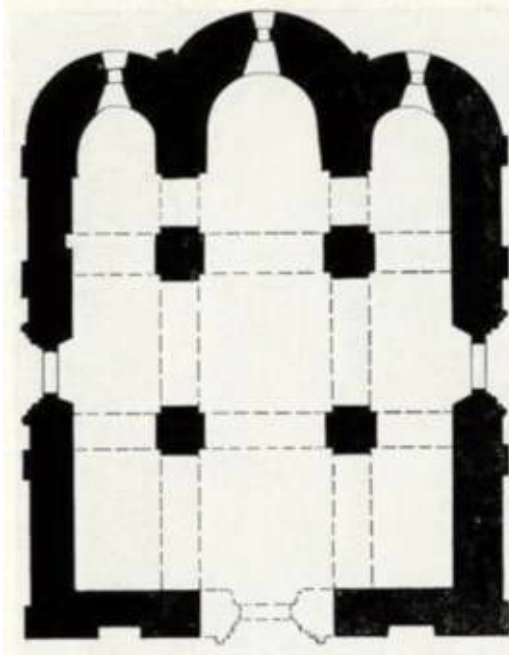
20. Архангельский собор. План
