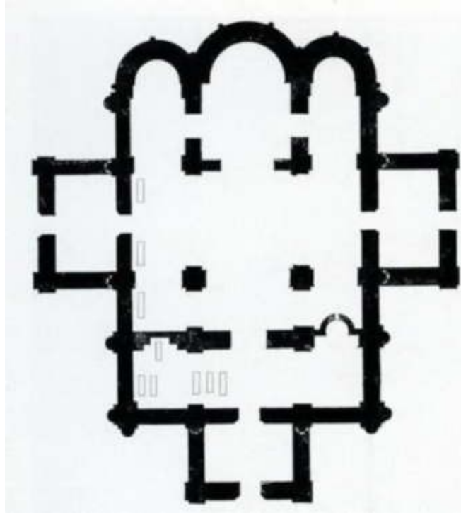
10. Успенский собор в Старой Рязани, ок. 1096 – 98. План. Реконструкция Е. Михайловского
