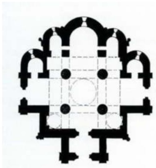
11. Спасский собор в Старой Рязани. XII в. План. Реконструкция Е. Михайловского
