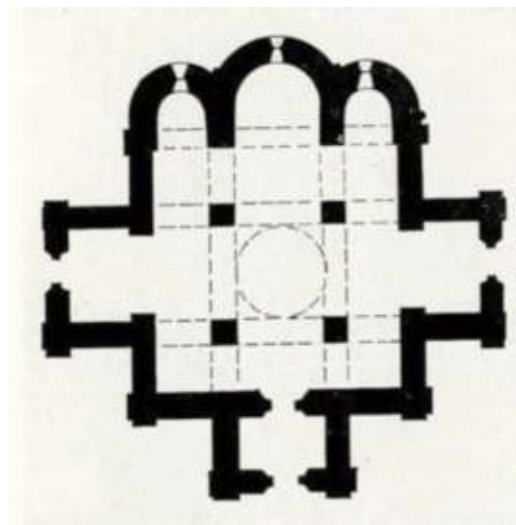
21. Старый Успенский собор. План. Реконструкция Е. Михайловского
