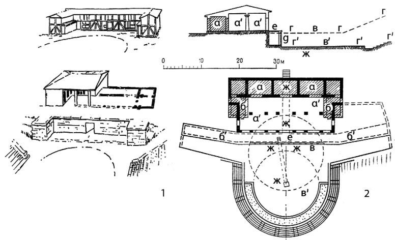
Развитие греческого театра (театр в Эретрии). 1 — первоначальный вид сцены и ее вид после перестройки (реконструкция); 2 — Устройство 4 в. до н. э. и перестройка 3-го в. до н. э.: а — сцена; б — парасцени; в — орхестра; г — уровень орхестры и уклон театра; а' — расширенная сцена; б' — пароды; в' — заглубленная орхестра; з' — уровень орхестры и уклон театра после перестройки; д — проскений; е — логейон; ж — подземные ходы (по В. Е. Быкову)
