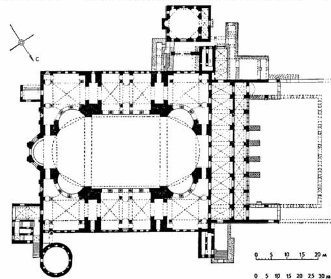
Собор св. Софии в Константинополе. Продольный разрез, план, по Н. И. Брунову
