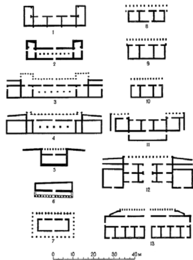
Планы сцен некоторых греческих театров: развитие проксения (по В. Е. Быкову). 1 — Эретрия; 2 — Сегеста; 3 — Афины (театр Диониса); 4 — Эпидавр; 5 — Ороп; 6 — Мантинейя; 7 — Делос; 8 — Приена; 9 — Ассос; 10 — Милет; 11 — Магнесия на Меандре; 12 — Сикион; 13 — Эфес
