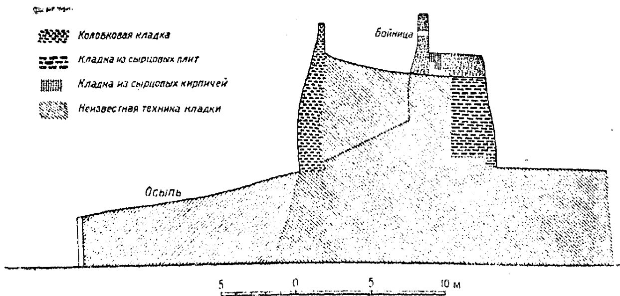
Рис. 4. Профиль башни и стены Ичан-Кала.
