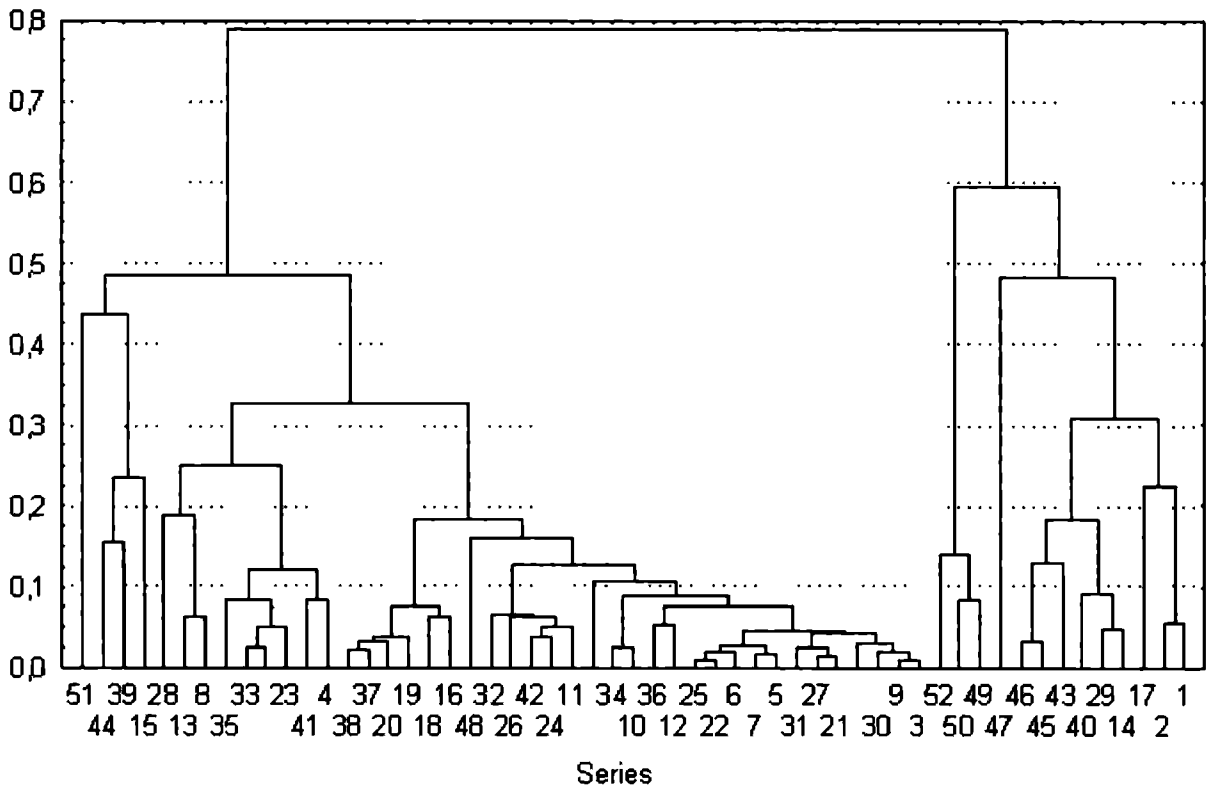
Рис. 7.9. Расположение исследованных групп по результатам кластерного анализа (по 11 признакам). Обозначение групп согласно нумерации в табл. 7.3
