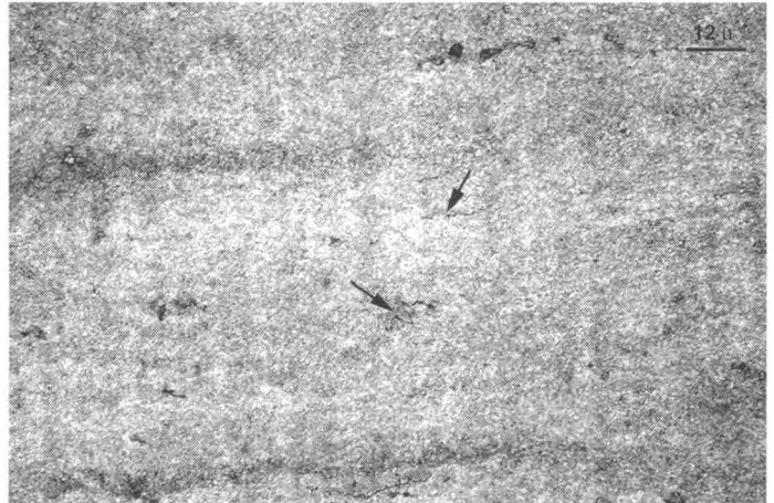
Рис. Пр.3.3. Деталь микроструктуры. Стрелки указывают на уплощенные халькоцитовые включения. Продукты травления те же, что и на рис. Пр. 3.2
