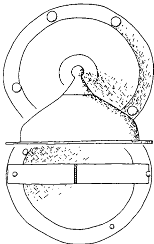
Рис. 48. Один из германских умбонов (тип Хорула), найденных в слоях разрушения 251 г. Танаис
