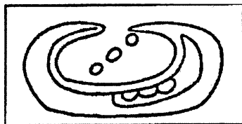
Рис. 108. Символ Луны
