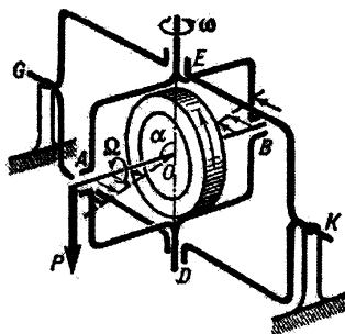
Рис. 67. Действие силы P на гироскоп с вращающимся ротором с тремя степенями свободы. Под воздействием этой силы ось вращения AB (Земли) будет смещаться в направлении, перпендикулярном направлению силы P , то есть перемещаться вокруг оси DE
