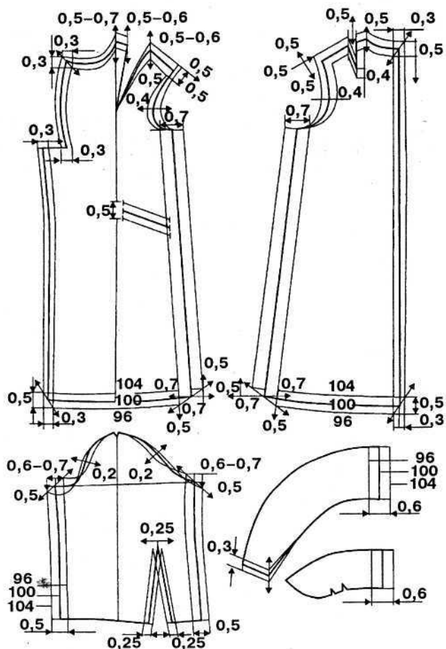
Рис. 31. Изменение размеров лекал деталей раскроя от размера 96 до 104
