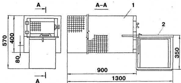
Рис. 13. Клетка для норок (размеры указаны в мм): 1 — выгул; 2 — домик
