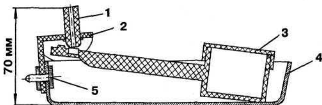
Рис. 30. Рычажно-поплавковая автопоилка:
