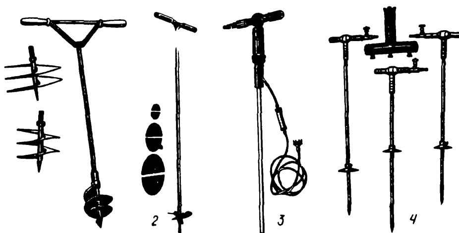
Рис. 121. Буры: 1 — шнековый; 2 — садовый; 3 — гидробур-растениепитатель; 4 — гидробур с распределителем ГБР (комплект).
