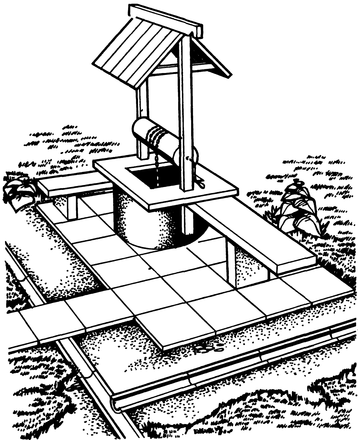
Рис. 6. Оформление питьевого колодца.
