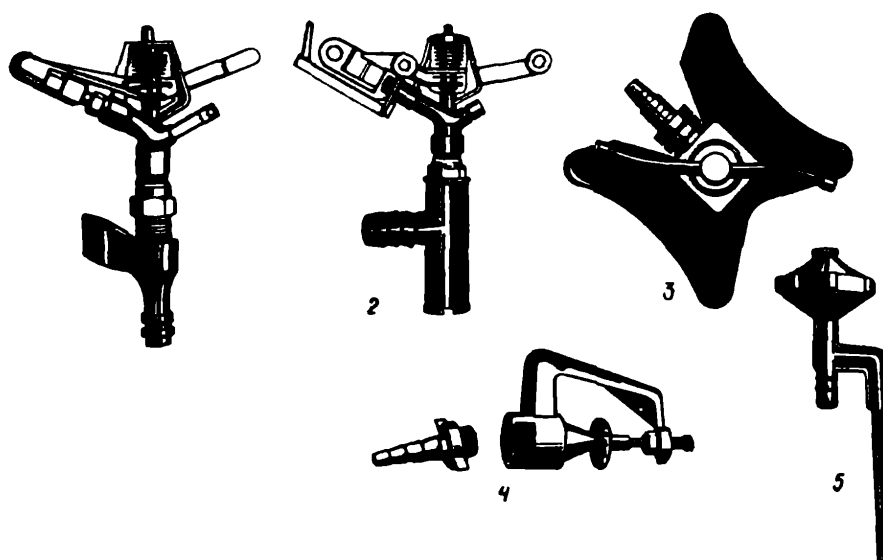
Рис. 119. Дождевальные аппараты: 1 — «Дождь»; 2 — АД-1; 3 — разбрызгиватель воды РВ-1; 4 — распыливатель воды РВО-8; 5 — распыливатель воды, регулируемый РВ.
