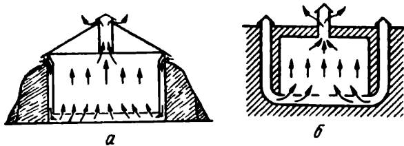
Рис. 142. Вентиляция в погребе: а — наземном; б — углубленном.
