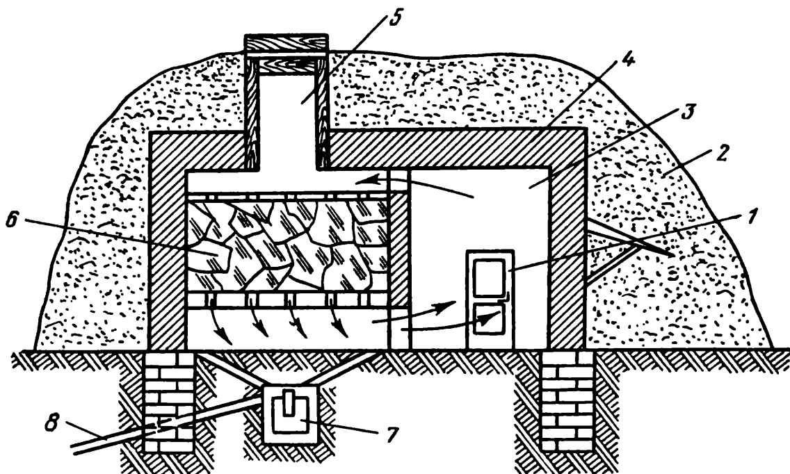
Рис. 143. Схема ледника с боковой загрузкой льда:
