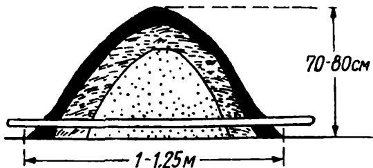
Рис. 57. Схема дымовой кучи.
